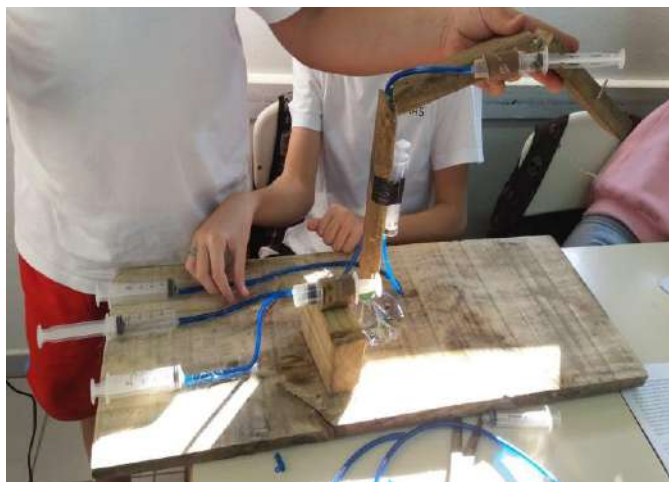
Figura 1 - Montagem do guindaste
