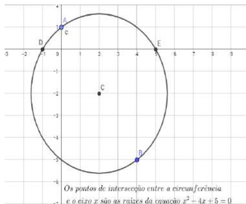
Figura 4: Construção completa do método de Thomas Carlyle
