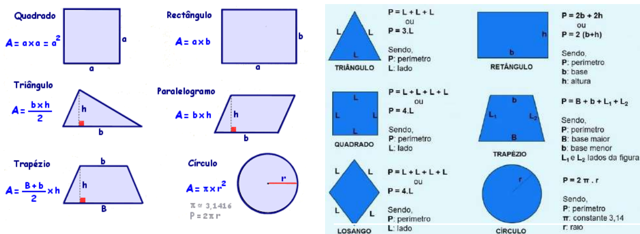
Figura 3.Área dos polígonos.
