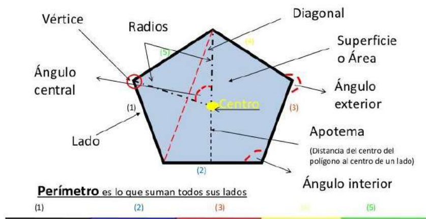
Figura 1- Elementos de um polígono
