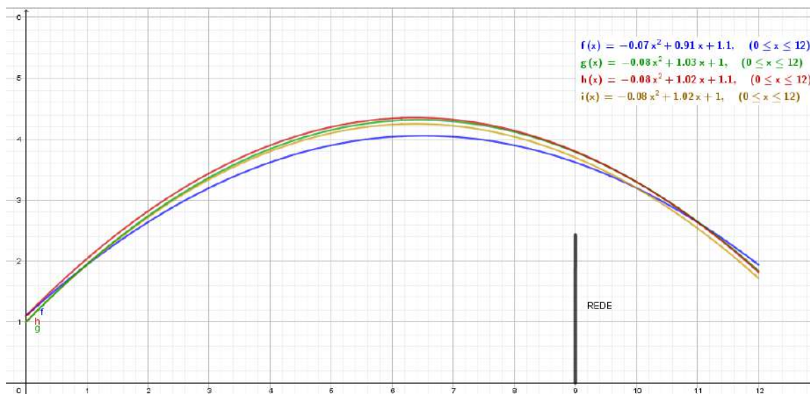
Imagem 5: Representação gráfica das funções no Geogebra.
