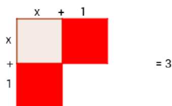
Figura 2: Transformar a figura em um quadrado
