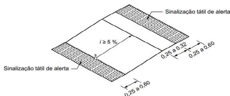
Figura 3 – piso tátil de alerta obrigatório para marcar lugares onde há desníveis, como rampas e escadas.
