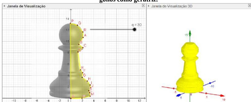
Figura 3: Interface de um dos simuladores, que permite a construção de sólidos de revolução usando polígonos como geratriz.
