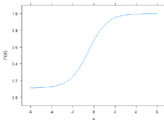
Figura 2 - Curva Característica do Item 137
