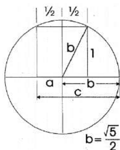
Figura 05: Diagrama da razão phi do corpo humano .
