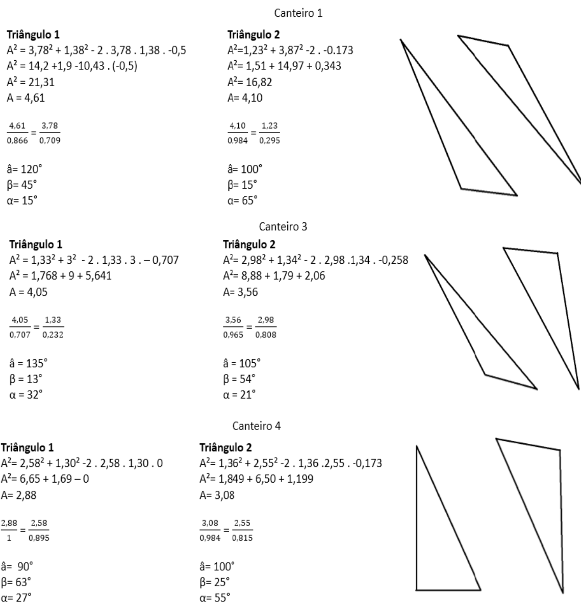
Figura 1 – Cálculos Trigonômicos.
