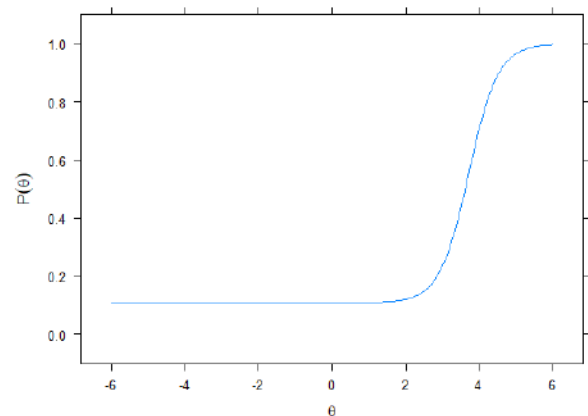
Figura 4 - Curva Característica do Item 162
