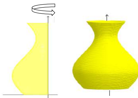
Figura 1: Sólido de revolução obtido pelo giro de um superfície plana sobre um eixo.
