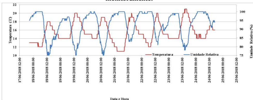
Figura 4 – Variação da temperatura e umidade relativa do ar ao longo de um dos períodos de monitoramento.
